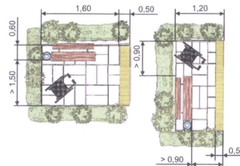
Зона отдыха для инвалидов
